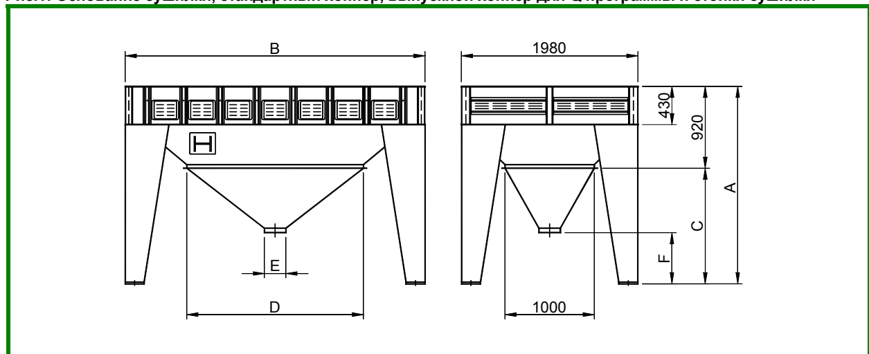
Рис.1: Основание сушилки, стандартный хоппер, выпускной хоппер для Q программы и стойки сушилки
